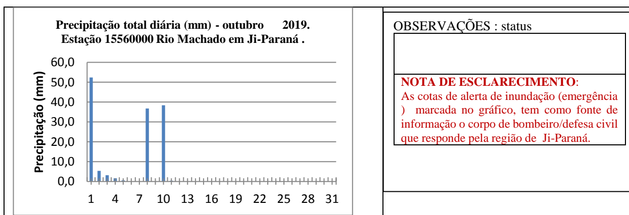
Gráfico 6.1- Monitoramento da precipitação total diária, na estação meteorológica Ji-Paraná – código 1061001, no rio Machado, em Ji-Paraná - RO.
