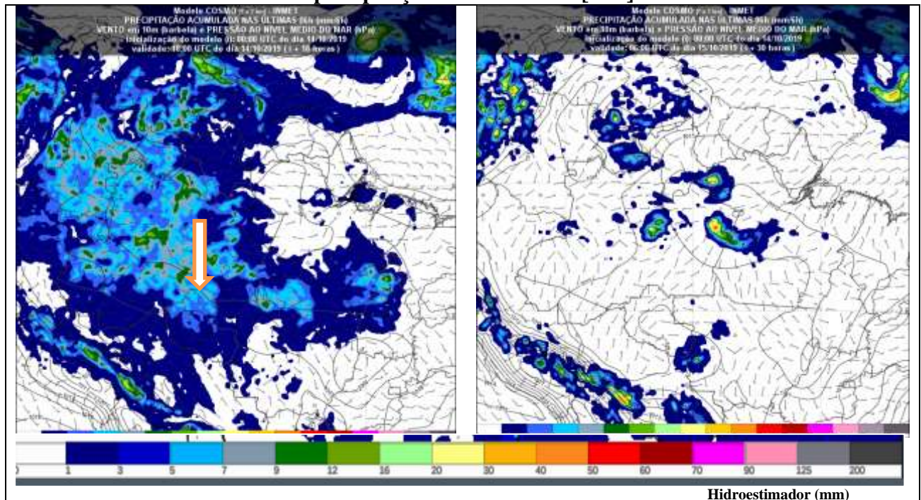
FIGURA 2 – Previsão do tempo no Estado de Rondônia para o dia 14/10/2019 as 18UTC
